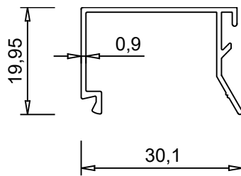
ALUM 1011 0.191 kg/m
