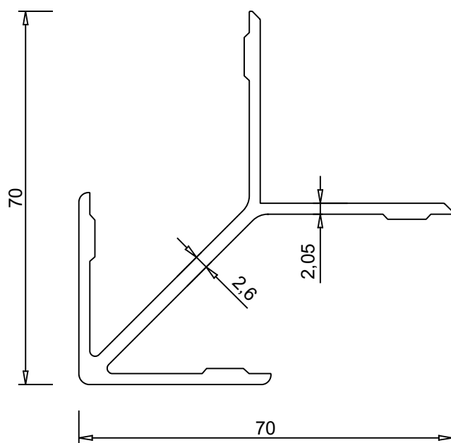
ALUM 1009 1.176kg/m
