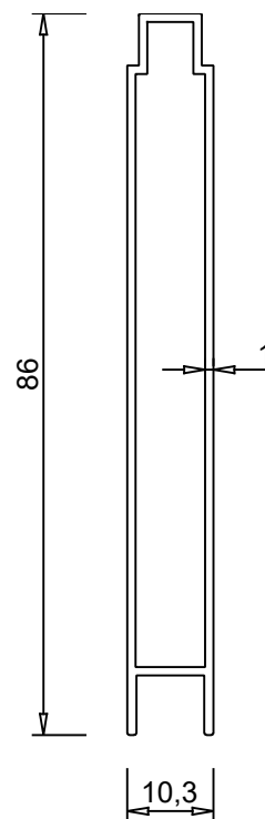
ALUM 1008 0.515 kg/m
