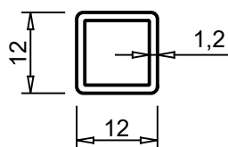
ALUM 2017 0.138 kg/m
