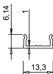
ALUM 2011 0.066 kg/m
