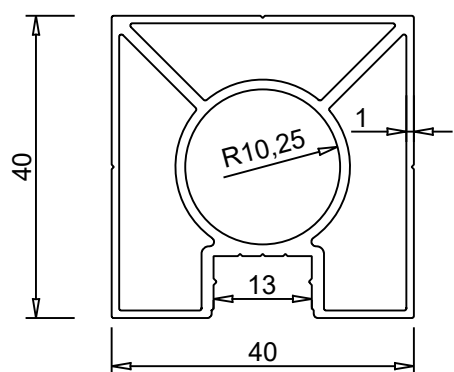
ALUM 2010 0.853 kg/m
