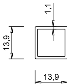
ALUM 2012 0.152 kg/m
