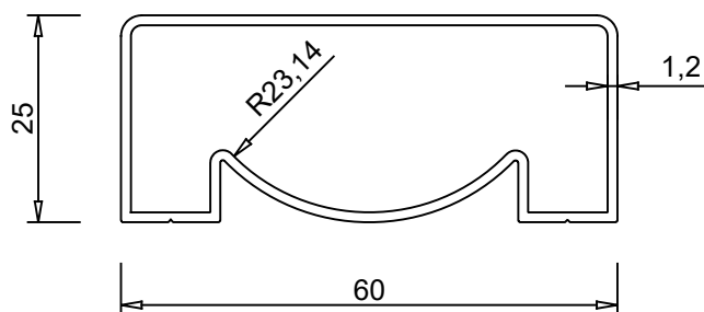
ALUM 2001 0.591 kg/m
