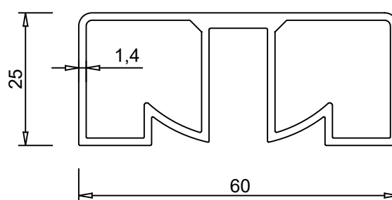
ALUM 2002 0.855 kg/m
