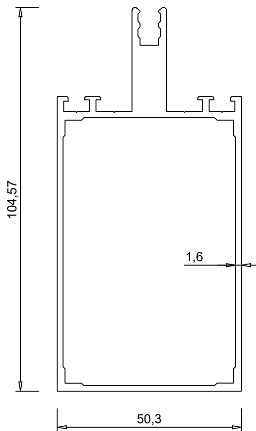
ALUM 5002 1.538 kg/m
