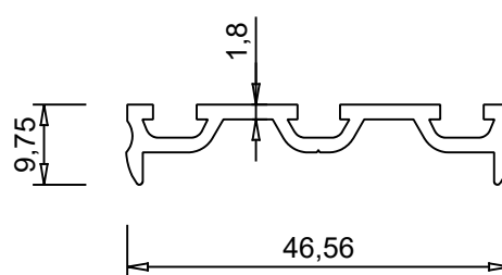
ALUM 5002 1.538 kg/m
