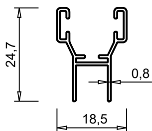
ALUM 10-005 0.173 kg/m
