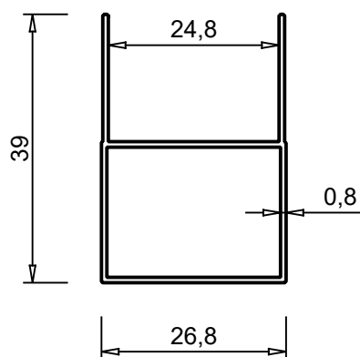
ALUM 10-008 0.279 kg/m
