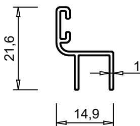
ALUM 10-006 0.138 kg/m
