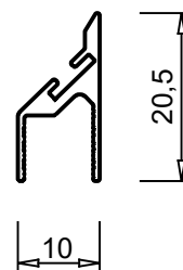
ALUM 10-007 0.136 kg/m
