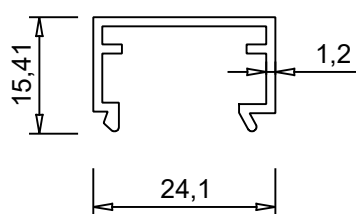
ALUM 3008 0.208 kg/m
