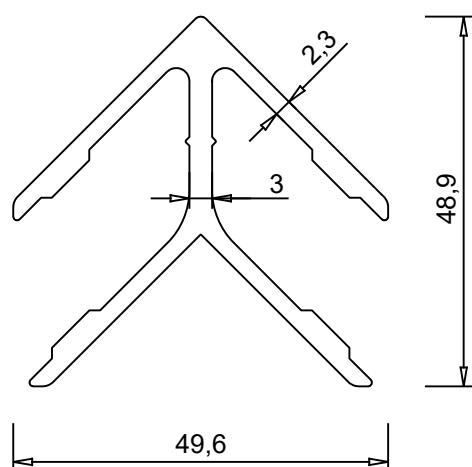
ALUM 3010 1.121 kg/m
