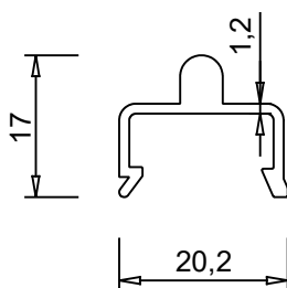
ALUM 3006 0.238 kg/m
