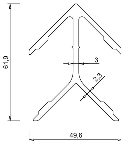
ALUM 3009 1.226 kg/m
