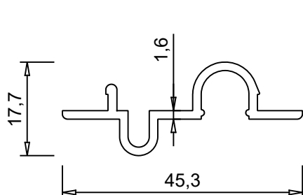
ALUM 3005 0.333 kg/m
