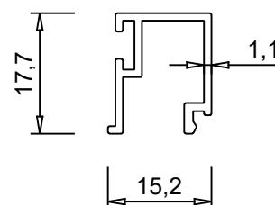
ALUM 3007 0.176 kg/m
